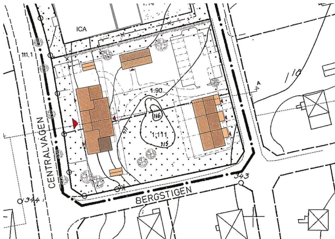
Figur 2. Skiss över möjlig exploatering på fastigheterna Prästgården 1:90 och Prästgården 1:111. Flerbostadshus mot Centralvägen samt radhuslänga mot Vätterbostigen. Skiss ateljé Wiggård arkitektur.
